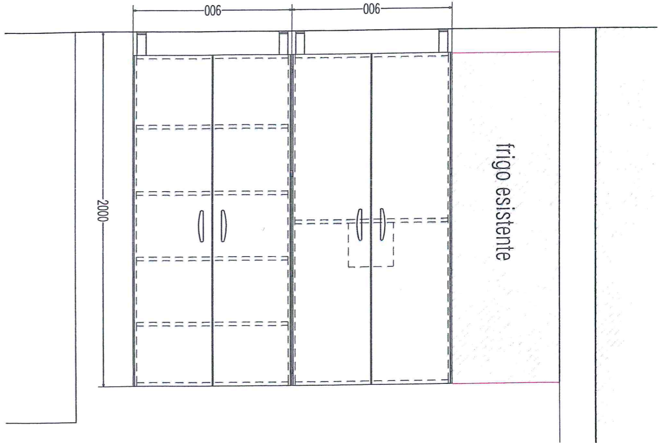
5 Parete Alta con Armadio Farmaci e colonna a ripiani SCALA 1:25
