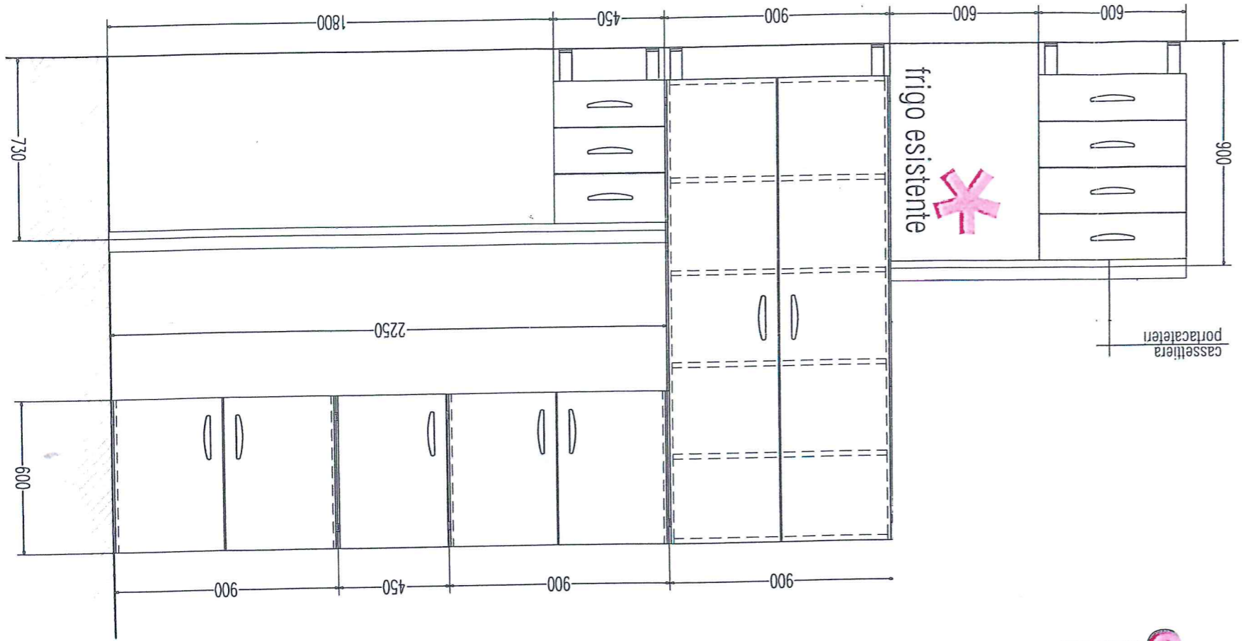
6 Parete bassa con basi e pensili SCALA 1:25
